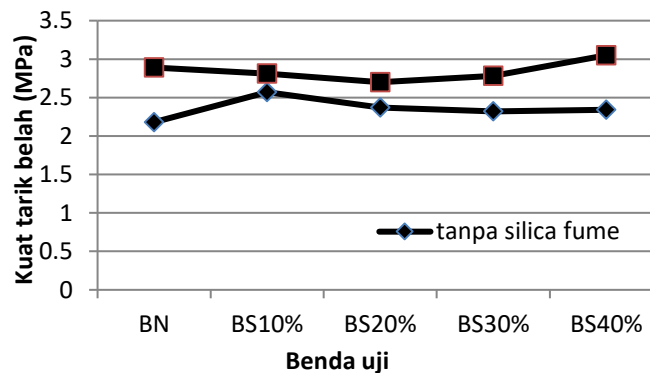
Gambar 11. Perbandingan kuat tarik belah
