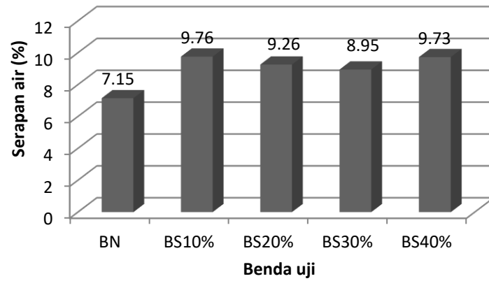
Gambar 13. Serapan air dengan silica fume
