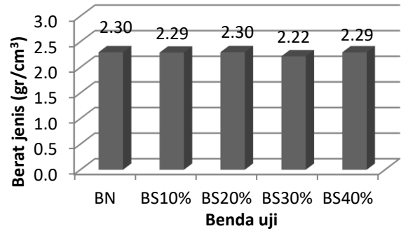
Gambar 2. Berat Jenis beton dengan silica fume
