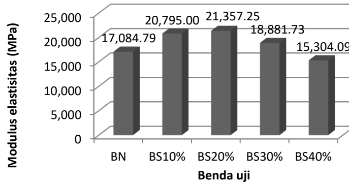
Gambar 6. Modulus elastisitas beton tanpa silica fume
