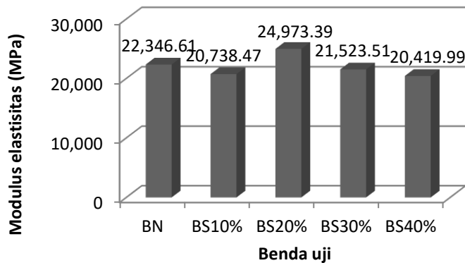
Gambar 7. Modulus elastisitas beton dengan silica fume
