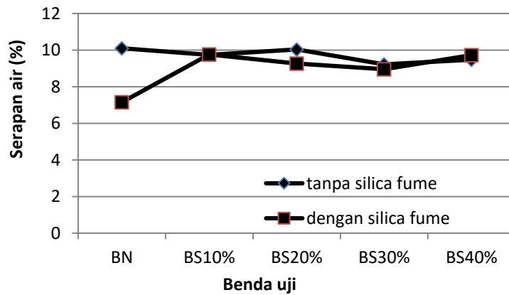
Gambar 14. Perbandingan serapan air
