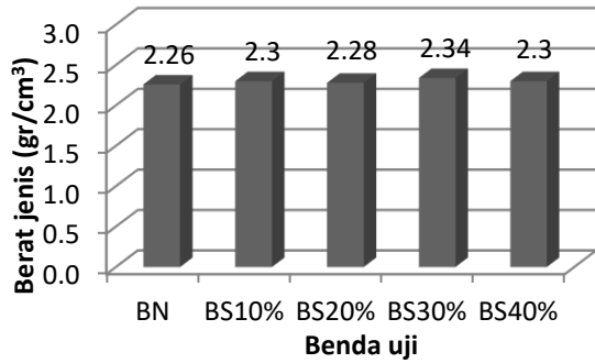
Gambar 1. Berat jenis beton tanpa silica fume
