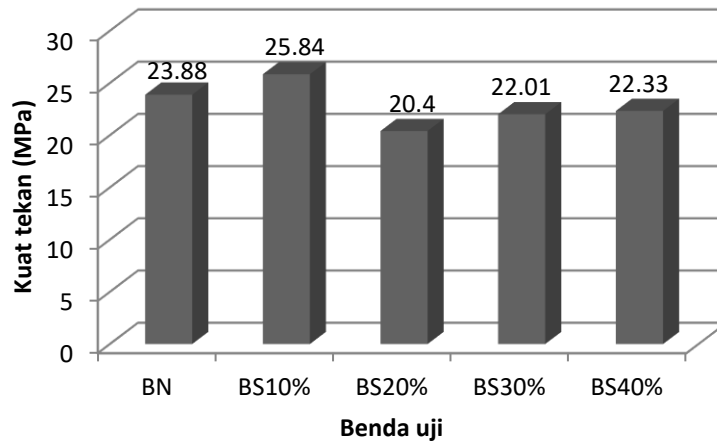
Gambar 3. Kuat tekan beton tanpa silica fume
