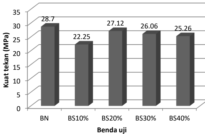
Gambar 4. Kuat tekan beton dengan silica fume
