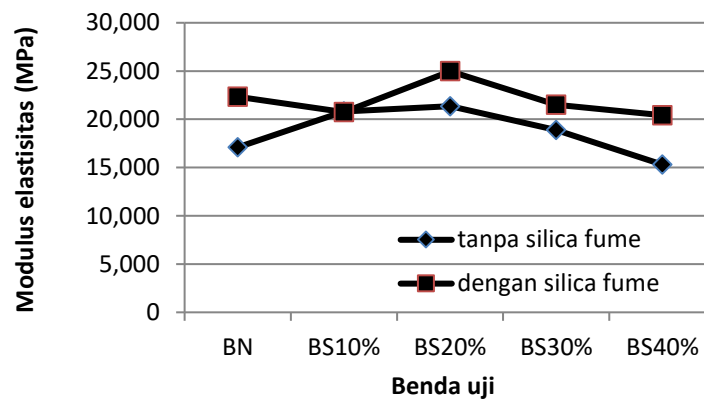
Gambar 8. Perbandingan modulus elastisitas
