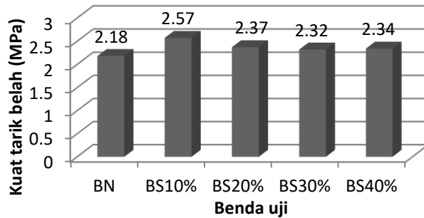
Gambar 9 Kuat tarik belah beton tanpa silica fume
