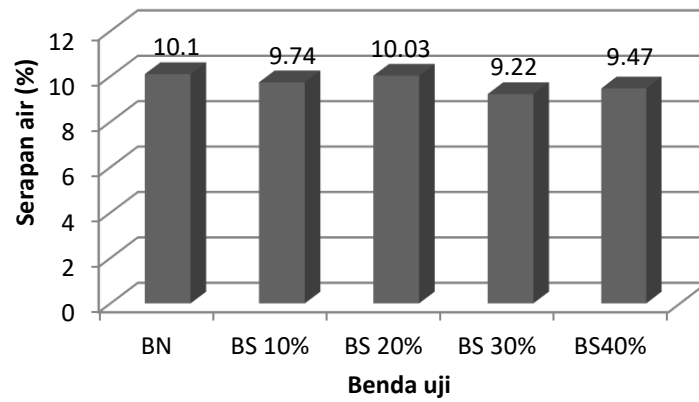
Gambar 12. Serapan air tanpa silica fume
