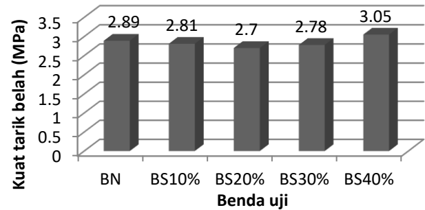
Gambar 10. Kuat tarik belah beton dengan silica fume
