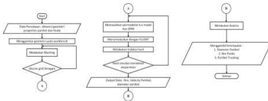
Gambar 2. Flowchart simulasi deposisi aerosol partikel
