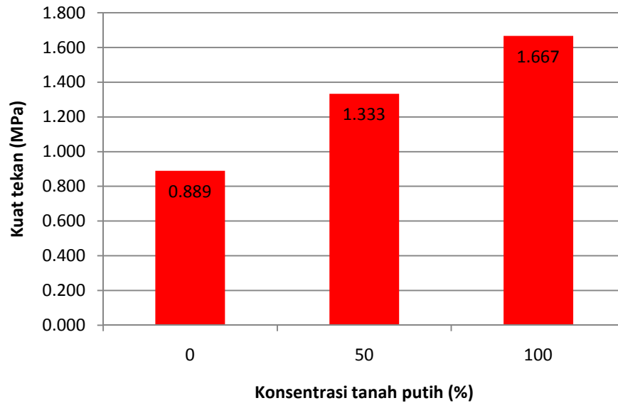
Gambar 5 Grafik Hubungan Antara Kuat Tekan Bata Ringan CLC Terhadap Konsentrasi Substitusi Tanah Putih Dalam Campuran Bata Ringan CLC pada Umur 14 Hari.
