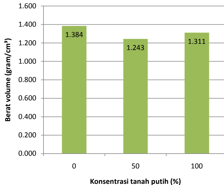
Gambar 3 Grafik Hubungan Antara Berat Volume Terhadap Konsentrasi Substitusi Tanah Putih Dalam Campuran Bata Ringan CLC pada Umur 28 Hari
