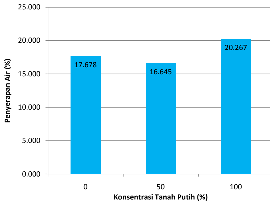
Gambar 7 Grafik Hubungan Antara Serapan Air Bata Ringan CLC Terhadap Konsentrasi Substitusi Tanah Putih Dalam Campuran Bata Ringan CLC pada Umur 28 Hari.
