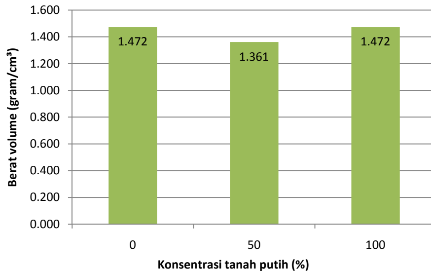
Gambar 6 Grafik Hubungan Antara Kuat Tekan Bata Ringan CLC Terhadap Konsentrasi Substitusi Tanah Putih Dalam Campuran Bata Ringan CLC pada Umur 28 Hari.
