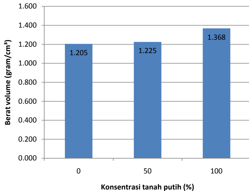
Gambar 1. Grafik Hubungan Antara Berat Volume Terhadap Konsentrasi Substitusi Tanah Putih Dalam Campuran Bata Ringan CLC pada Umur 7 Hari.
