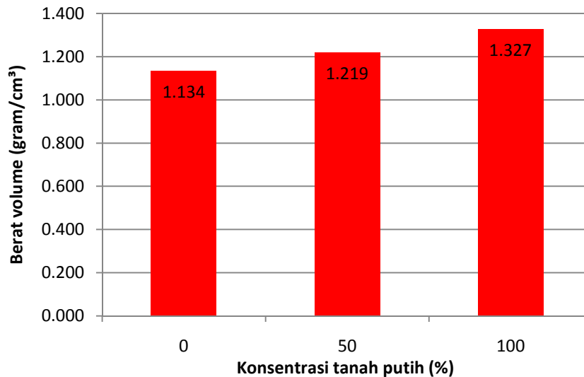
Gambar 2. Grafik Hubungan Antara Berat Volume Terhadap Konsentrasi Substitusi Tanah Putih Dalam Campuran Bata Ringan CLC pada Umur 14 Hari.
