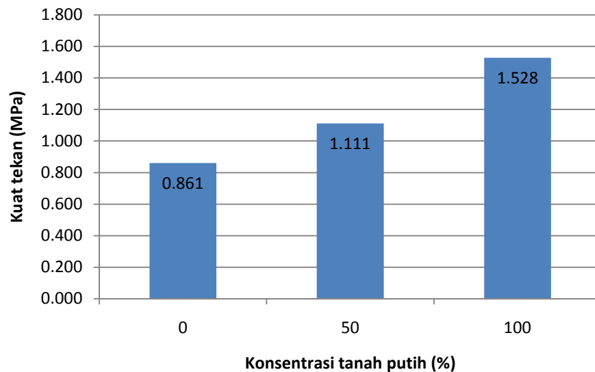
Gambar 4 Grafik Hubungan Antara Kuat Tekan Bata Ringan CLC Terhadap Konsentrasi Substitusi Tanah Putih Dalam Campuran Bata Ringan CLC pada Umur 7 Hari.
