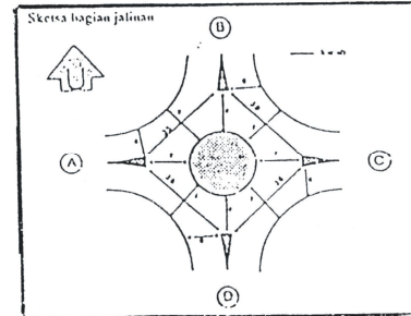
Gambar Sketsa Masukan Geometri (Sumber: MKJI, 1997)
