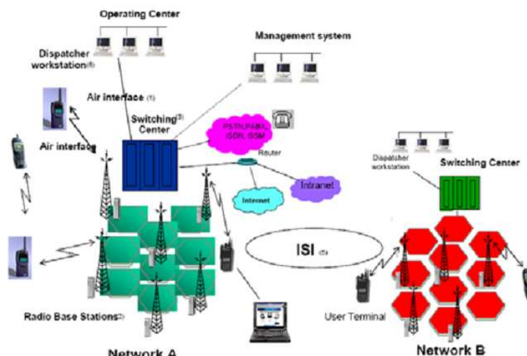
Gambar 2. Arsitektur TETRA
