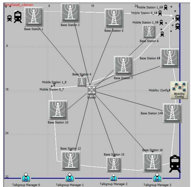
Gambar 8. Topologi jaringan TetraDaop8 20 node
