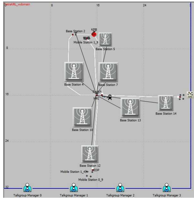
Gambar 6. Topologi jaringan TetraKRL 20 node
