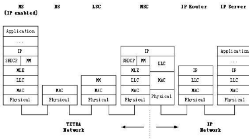
Gambar 4. Peer to peer untuk interworking TETRA dengan internet
