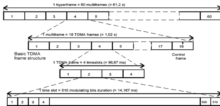
Gambar 3. Struktur Frame TDMA TETRA
