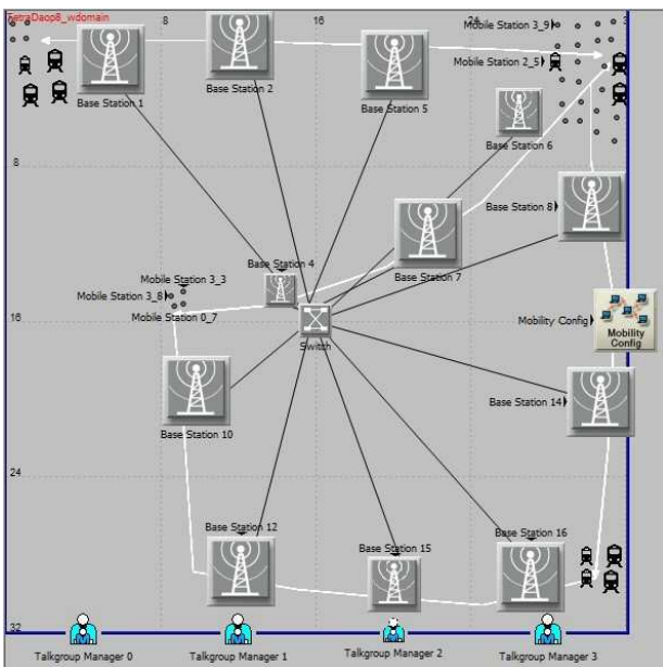
Gambar 7. Topologi jaringan TetraDaop8 40 node
