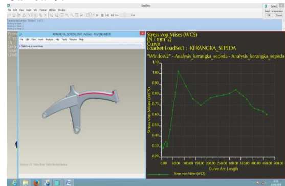
Gambar 9. Analisis grafik tegangan Von Mises terhadap rangka sepeda komposit
