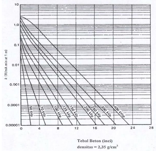
Gambar. 2. Grafik Faktor Pelemahan Sinar-X [7]
