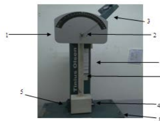
Gambar 7. Alat pengujian ketangguhan
