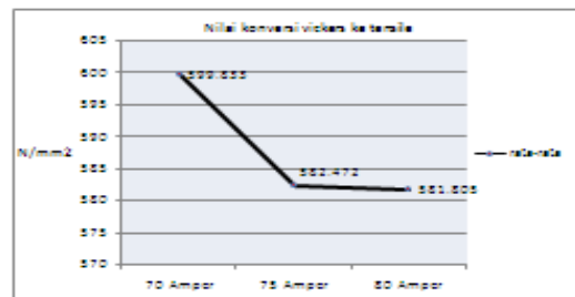
Gambar 21 Grafik Nilai Rata-rata Hasil Konversi Vickers ke Tensile strength
