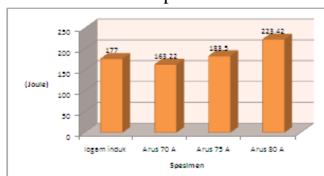
Gambar 15. Hasil pengujian tes impact arus 80 Amper.
