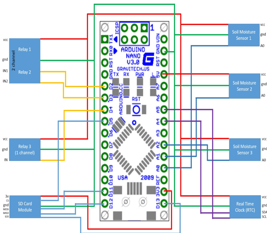
Gambar 1. Rancangan Sistem Kendali Otomatis
