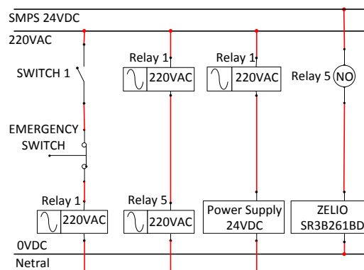
Gambar 7 Rangkaian relay untuk mengaktifkan Zelio
