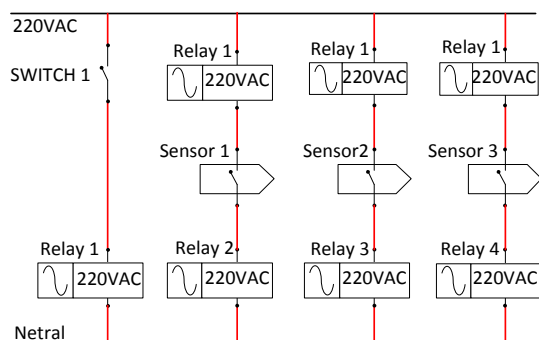
Gambar 5 Rangkaian relay untuk sensor
