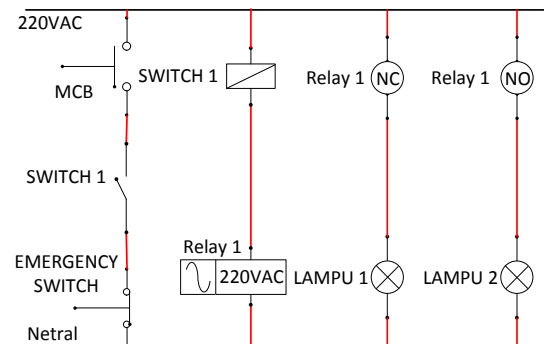
Gambar 4 Rangkaian switch
