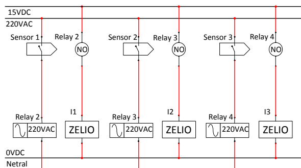
Gambar 6 Output sensor sebagai input Zelio
