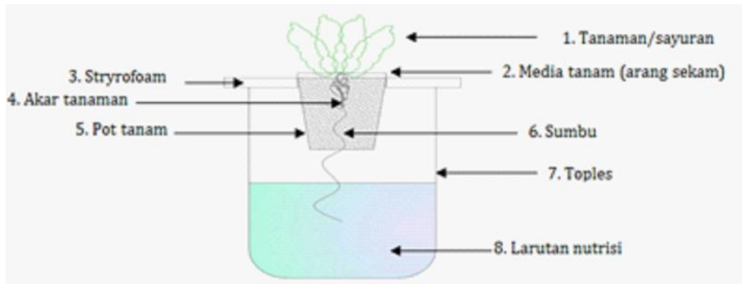
Gambar 1. Sistem Hidroponik Sumbu
