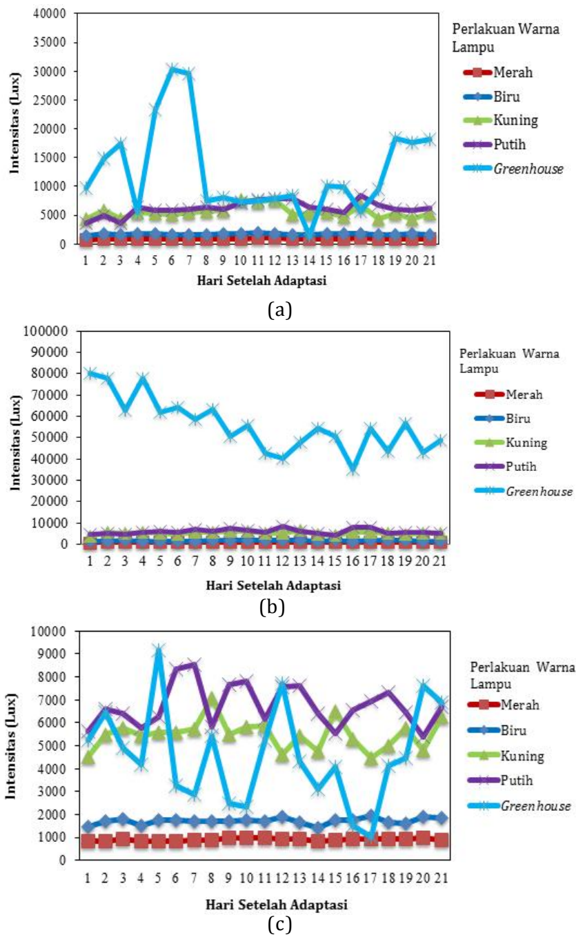
Gambar 3. Intensitas Cahaya Pada (a) Pagi Hari, (b) Siang Hari, dan (c) Sore Hari
