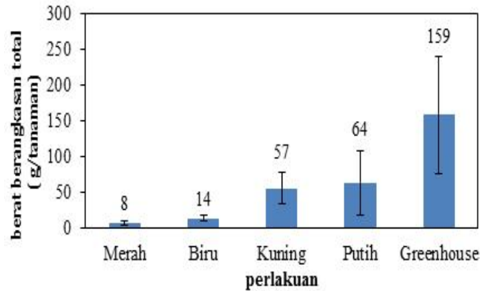
Gambar 11. Pengaruh Penggunaan Warna Lampu Neon Terhadap Berat berangkasan total Kailan
