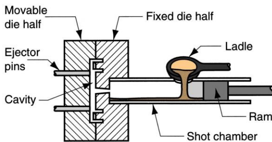
Gambar 3. Mesin HPDC[6].
