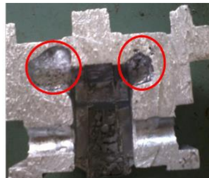
Gambar 12. Shrinkage pada temperatur cetakan 350°C
