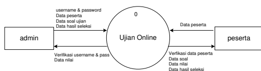
Gambar 3.2 Konteks Diagram
