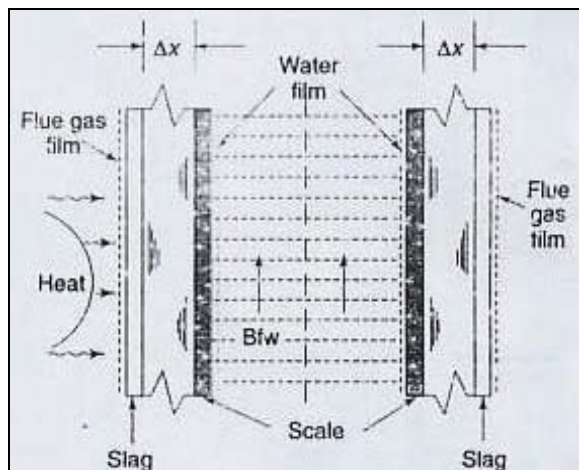
Gambar 6. Modus Perpindahan di dalam Boiler [6]
