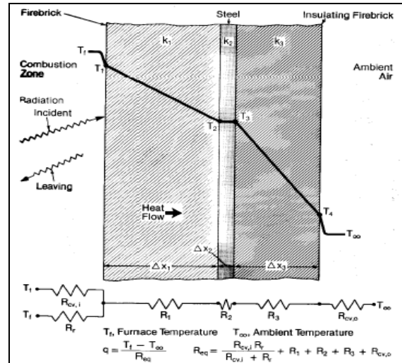
Gambar 7. Mekanisme Kehilangan Kalor pada Dinding Ruang Bakar [9]
