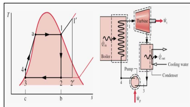
Gambar 3. Siklus Rankine Sederhana [2]
