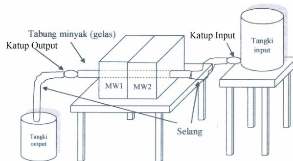
Gambar 1. Perangkat Transesterifikasi
