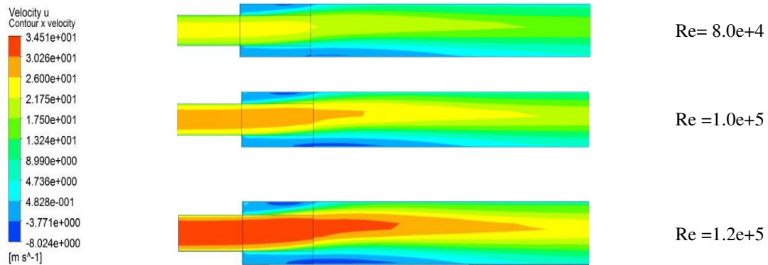
Gambar 8. Hasil simulasi kontur x-velocity
