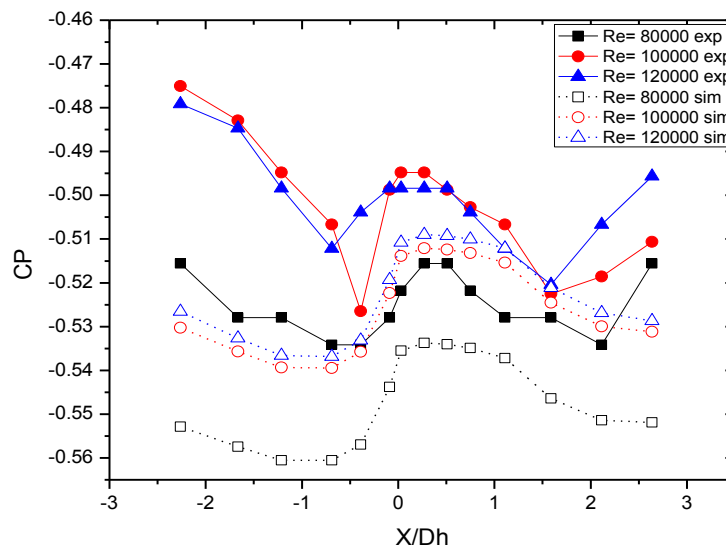
Gambar 5. Distribusi C_p pada Y/Dh = -0.72
