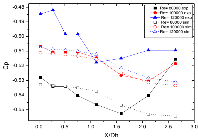
Gambar 6. Distribusi C_p pada Y/D_h = -1.28
