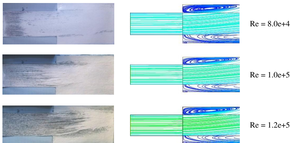
Gambar 9. Perbandingan streamline hasil eksperimen dan simulasi numerik
