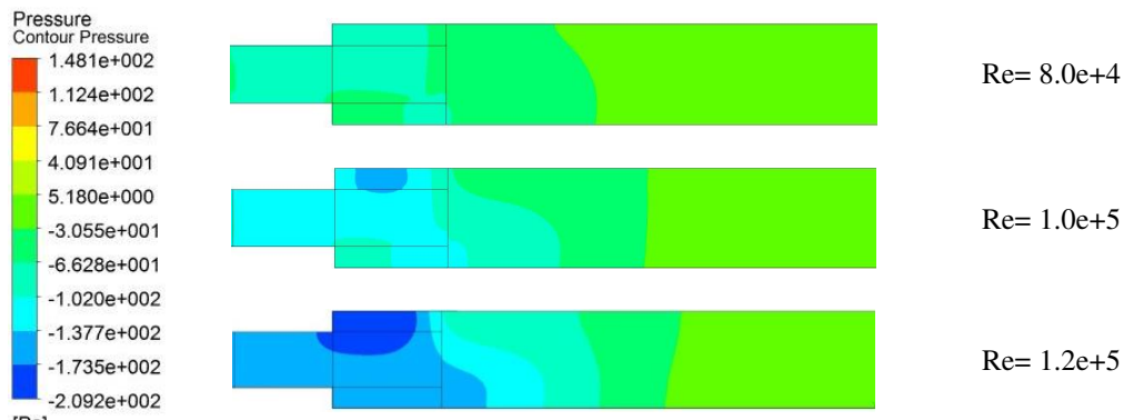
Gambar 7. Hasil simulasi kontur distribusi tekanan statis
