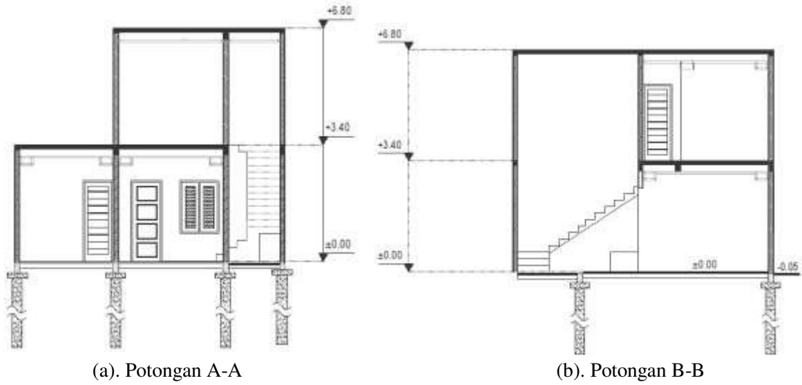
Gambar 4. Potongan A-A dan Potongan B-B (elevasi dalam satuan meter)
