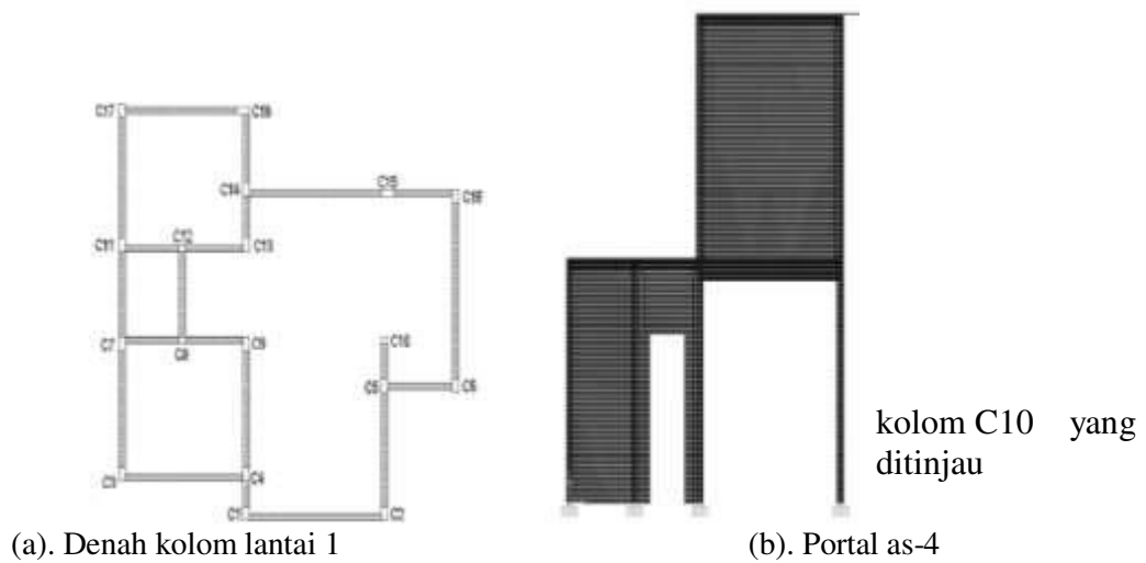
Gambar 12. Kolom C10 yang ditinjau
