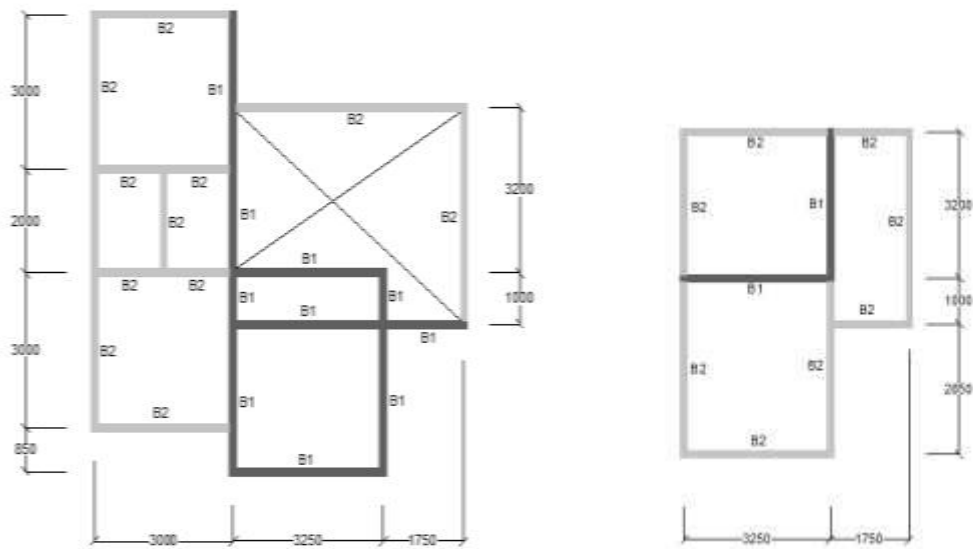
Gambar 5. Denah pembalokan lantai 1 dan lantai 2 (unit satuan cm)
