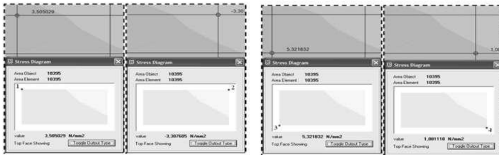
Gambar 11. Kontur tegangan normal ( S_{11} ) pada balok B7
