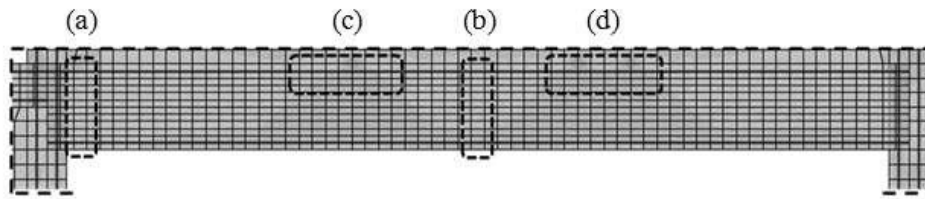
Gambar 10. Hasil simulasi numerik, Tegangan S_{11} pada balok B7
