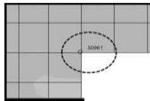
Gambar 18. Hasil analisis berupa kontur tegangan pada kusen pintu yang ditinjau.
