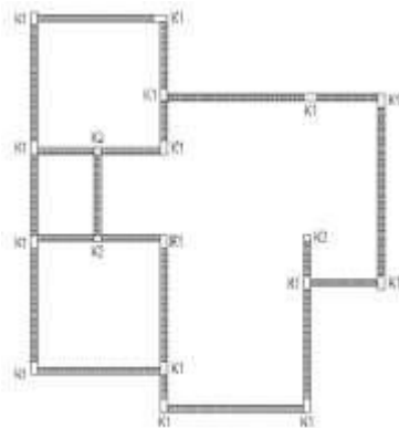
Gambar 6. Denah kolom lantai 1
