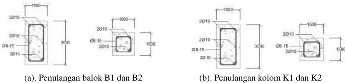
Gambar 7. Detail penulangan balok dan kolom (unit satuan mm)
