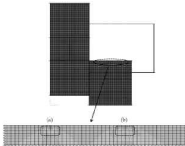
Gambar 15. Kontur tegangan pada pelat lantai
