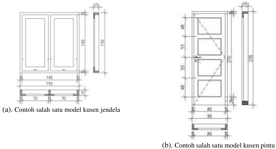
Gambar 8. Contoh salah satu model kusen jendela dan pintu (unit satuan cm)
