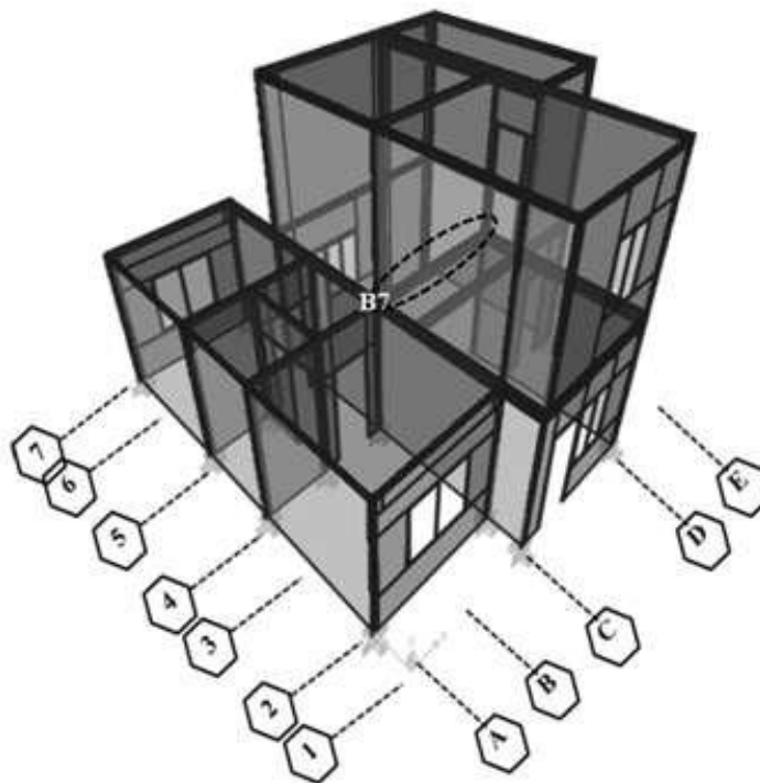
Gambar 9. Skematik model 3D bangunan dengan metode elemen hingga
