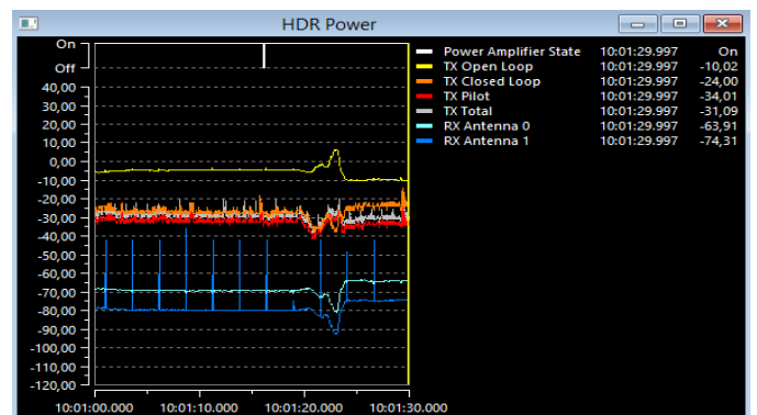
Gambar 15. Kuat sinyal setelah menggunakan antenna
