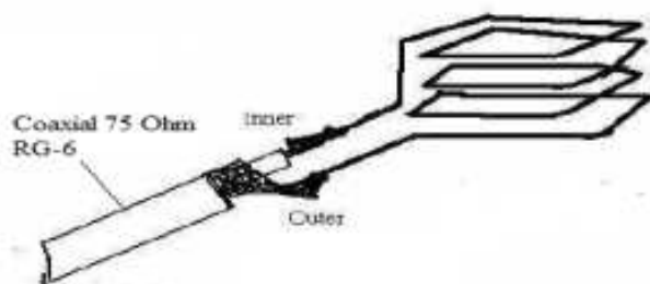
Gambar 6. Induksi lilitan kabel
