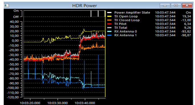
Gambar 13. Kuat sinyal sebelum menggunakan antenna
