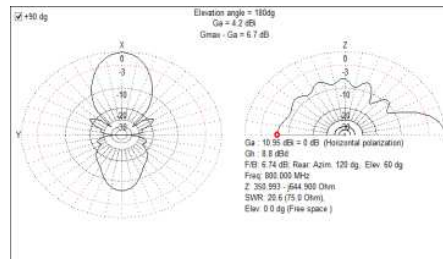
Gambar 7. Simulasi sebelum dimodifikasi
