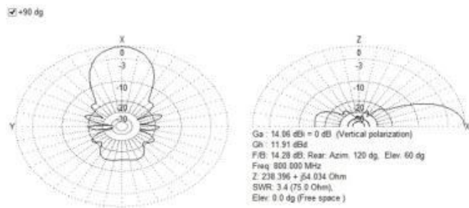
Gambar 9. Simulasi setelah modifikasi
