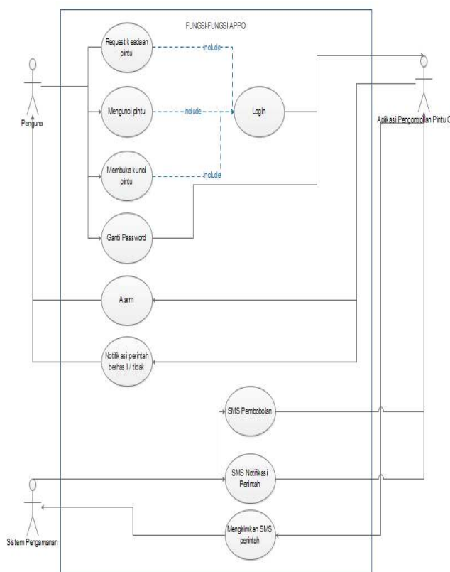
Gambar 4. Use case diagram fungsi dari APPO
