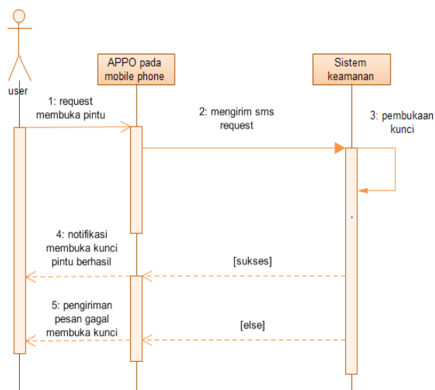
Gambar 8. Sequence diagram fitur membuka kunci pintu
