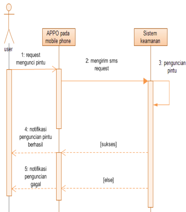
Gambar 7. Sequence diagram fitur mengunci pintu
