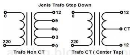
Gambar 2.7 Trafo step down
