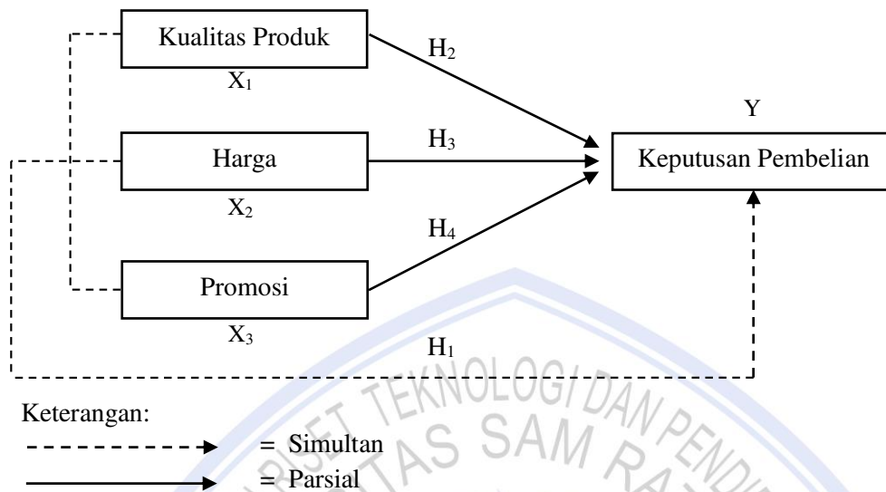
Gambar 2. Kerangka Konseptual
