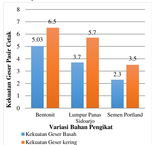
Diagram 2. Perbandingan Kekuatan Geser Pasir Cetak
