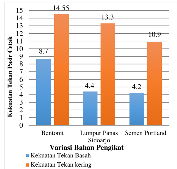
Diagram 1. Perbandingan Kekuatan Tekan Pasir Cetak
