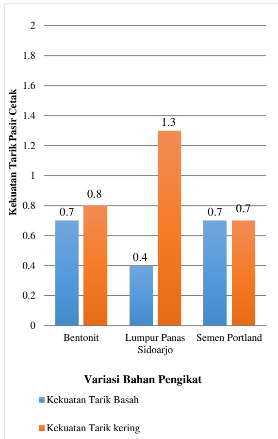
Diagram 3. Perbandingan Kekuatan Tarik Pasir Cetak
