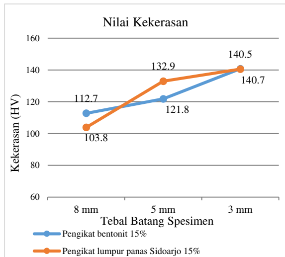
Diagram 5. Perbandingan Nilai Kekerasan HV terhadap Tebal Spesimen
