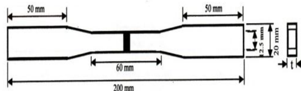
Gambar 3. Bentuk Pola uji tarik
