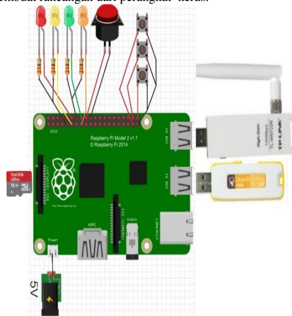
Gambar 16. Rancangan perangkat keras
