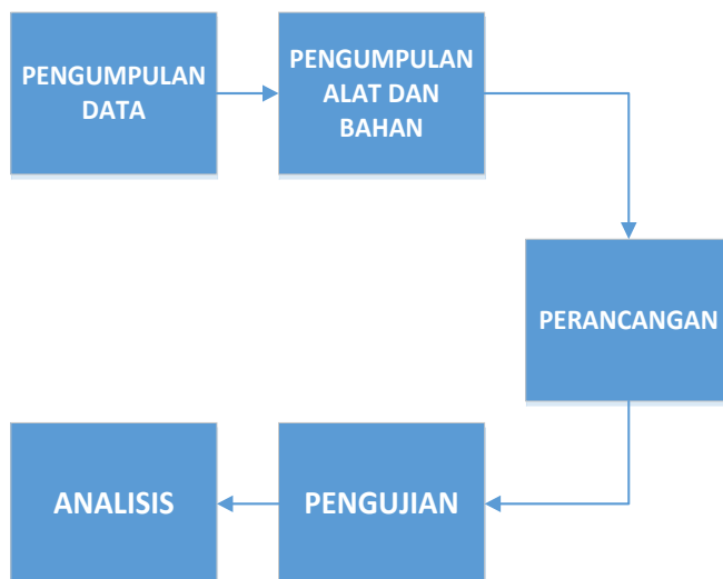
Gambar 14. Tahapan Penelitian
