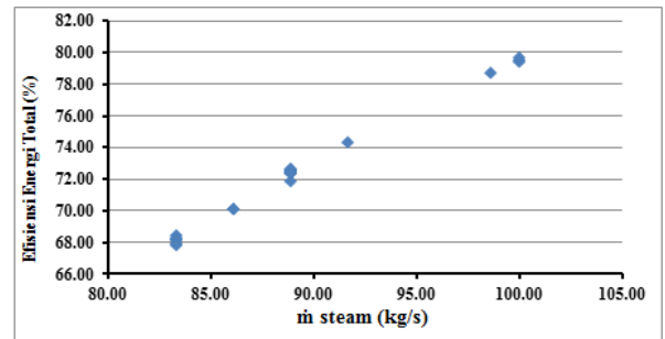
Gambar 6. Grafik pengaruh laju aliran massa steam terhadap efisiensi energi total boiler.
