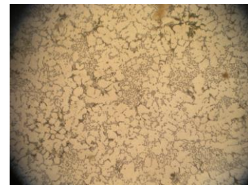
Gambar 5. Struktur Mikro Produk Sepatu Rem dengan Temperatur Penuangan 750°C
