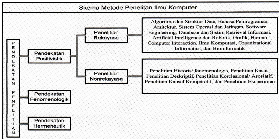
Gambar 1. Skema Klasifikasi Metodologi Penelitian Bidang IK
