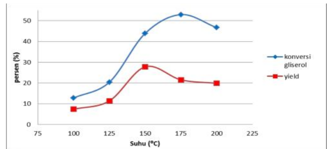
Gambar 4. Pengaruh suhu operasi terhadap konversi dan yield
