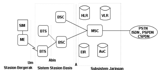
Gambar 2. Arsitektur jaringan GSM
