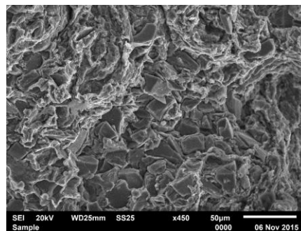
Gambar 11. Hasil SEM Spesimen uji tarik
