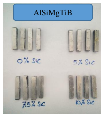
Gambar 6. Spesimen uji impact
