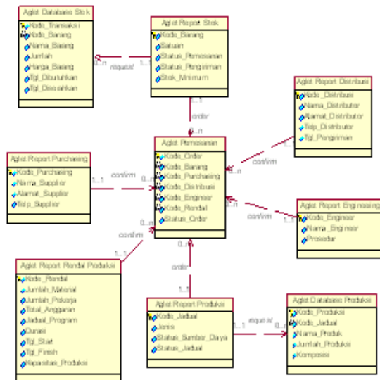
Gambar 12 Basis Data untuk Server PT. TNF
