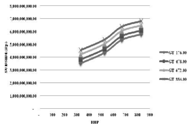
Gambar. 3. Besarnya Subsidi dengan Perubahan BHP Kapal.
