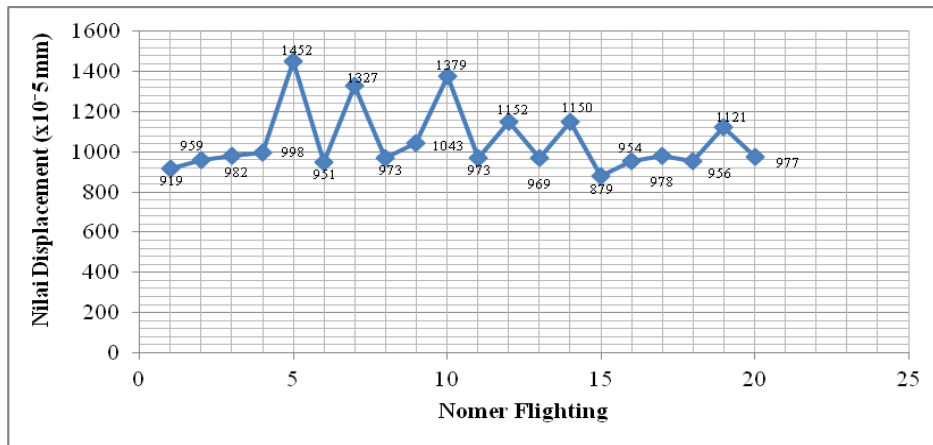
Gambar 7. Grafik perbandingan nilai displacement maksimal pada daun screw 1-20.
