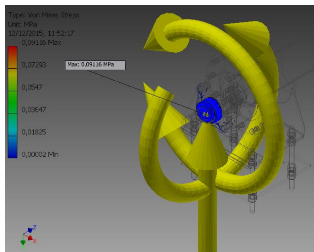
Gambar 5. Beban dinamis pada bearing .
