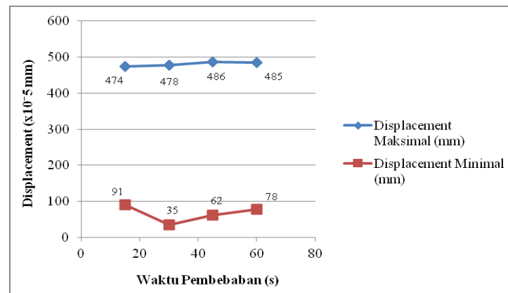
Gambar 12. Grafik perbandingan nilai displacement pada bearing .
