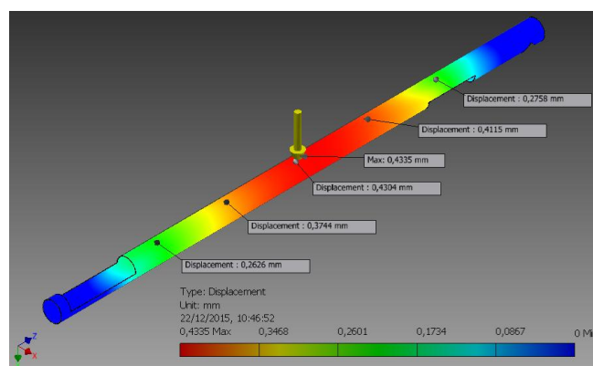
Gambar 8. Pandangan isometrik analisa kelendutan chasing screw sebelum terisi material.
