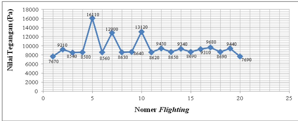
Gambar 6. Grafik perbandingan nilai tegangan maksimal pada parameter von mises stress pada daun screw 1-20.
