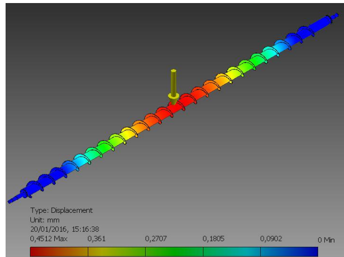
Gambar 10. Pandangan isometrik analisa kelendutan.
