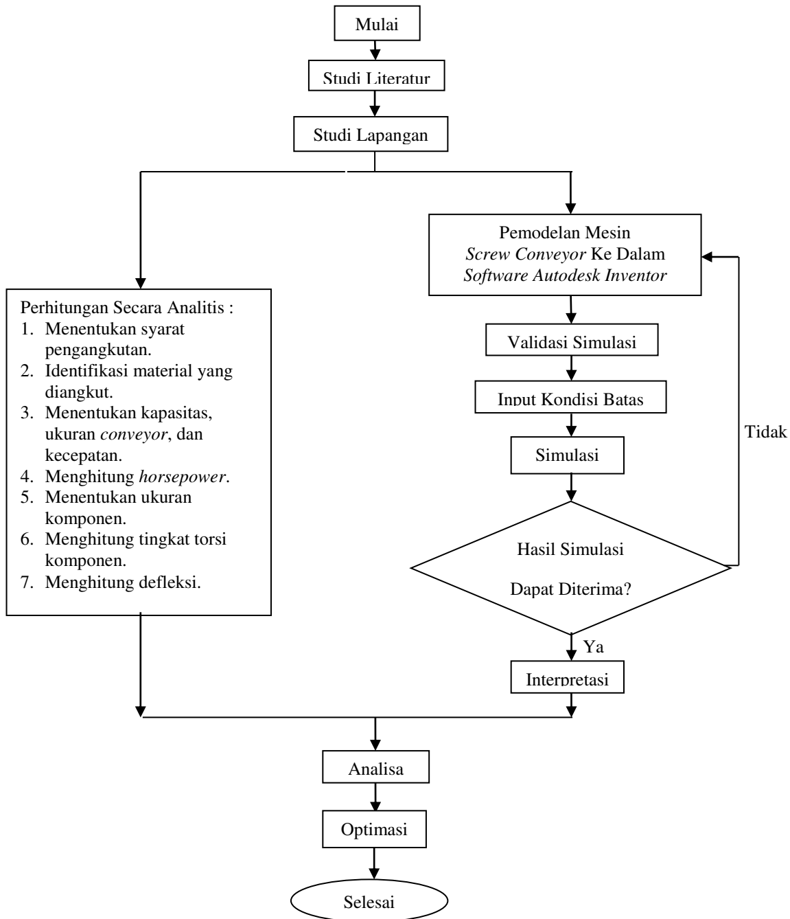
Gambar 1. Diagram alir pengujian
