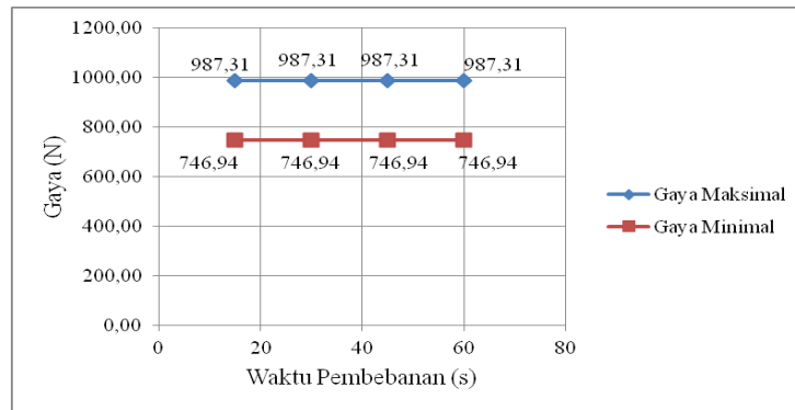
Gambar 10. Grafik perbandingan gaya maksimal dan minimal simulasi dinamis.
