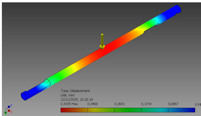
Gambar 3. Pengujian kelendutan chasing .
