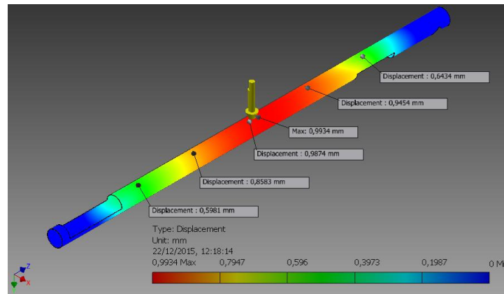
Gambar 9. Displacement pada setiap titik pemeriksaan chasing setelah terisi material.
