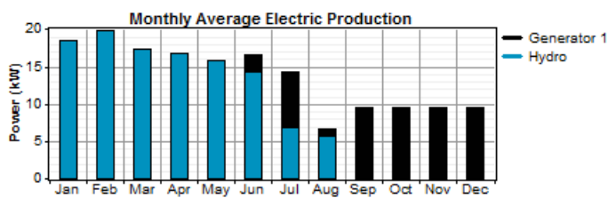
Gambar 5 Rata-rata produksi listrik per bulan
