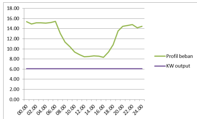
Gambar 3 Perbandingan daya keluaran bulan Agustus dan profil beban rata-rata desa Praingkareha
