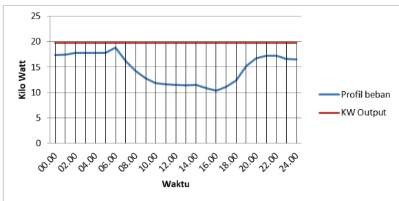
Gambar 1 Profil beban bulan Januari dan besar daya rata-rata yang diproduksi
