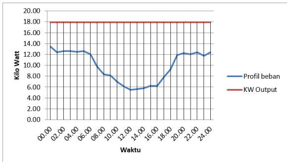
Gambar 2 Profil beban bulan April dan besar daya rata-rata yang diproduksi
