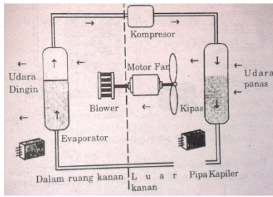
Gambar 1. Komponen kelistrikan peralatan AC
