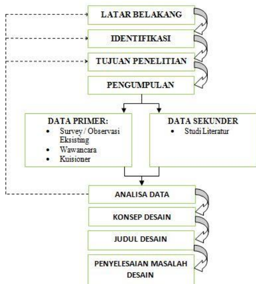
Gambar 2. Proses Desain
