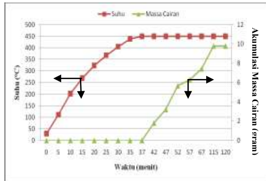
Gambar.8. Perolehan Massa Cairan yang Dihasilkan pada Pirolisis Sampah AL
