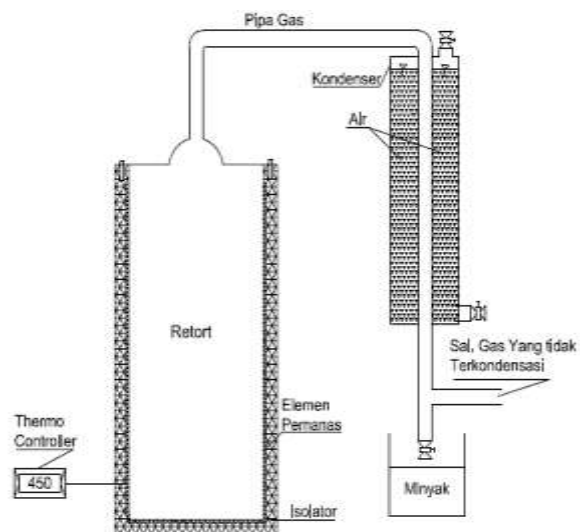
Gambar 2. Alat Pirolisis
