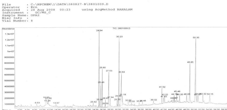
Gambar 3. Analisa GCMS (Gas Chromatography Mass Spektrofotometri) bahan aktif dari ekstrak handeuleum daun hijau corak putih dipinggir batang coklat ( G. pictum variagata alba )
