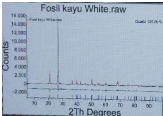
Gambar 6. Grafik Dikfragtogram XRD menunjukkan mineral penyusun fosil kayu 100% Quartz (Kuarsa)
