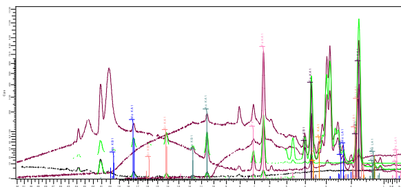
Gambar 7. Hasil analisa XRF yang menunjukkan senyawa penyusun fosil kayu senyawa terdiri \text{SiO}_2 90,84%, \text{Fe}_2\text{O}_3 3,95%, \text{CaO} 2,03% dan senyawa lainnya
