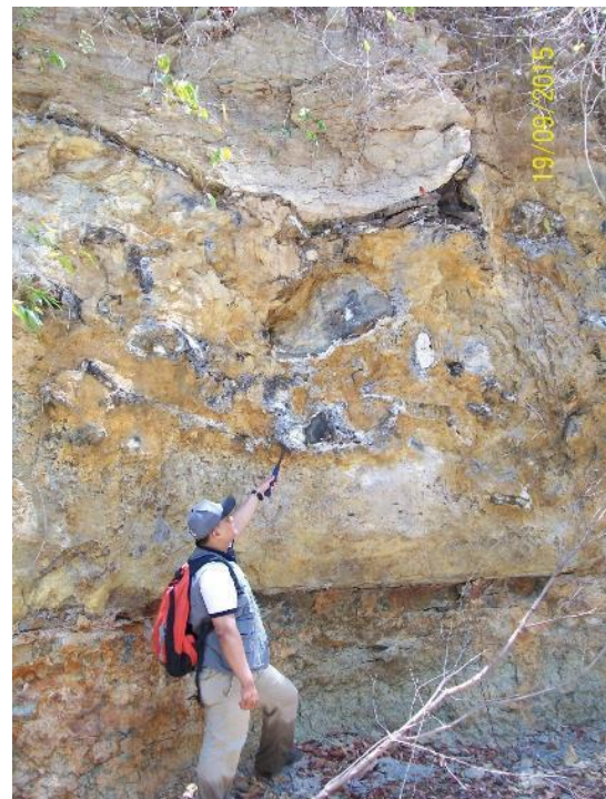
Gambar 3. Singkapan fosil kayu yang terdapat pada batupasir tufaan
