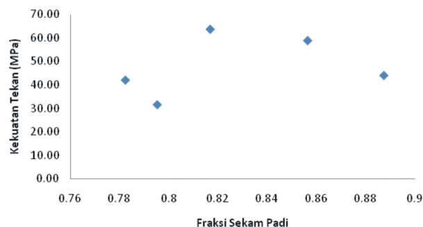
GAMBAR 1: Grafik kekuatan tekan terhadap fraksi sekam padi
