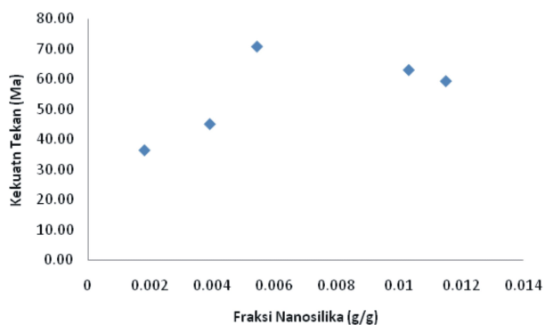
GAMBAR 2: Grafik kekuatan tekan terhadap fraksi nanosilika
