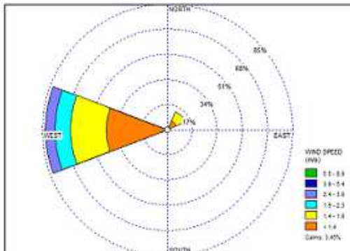
Gambar 4. Windrose musim Peralihan I (2003-2012)
