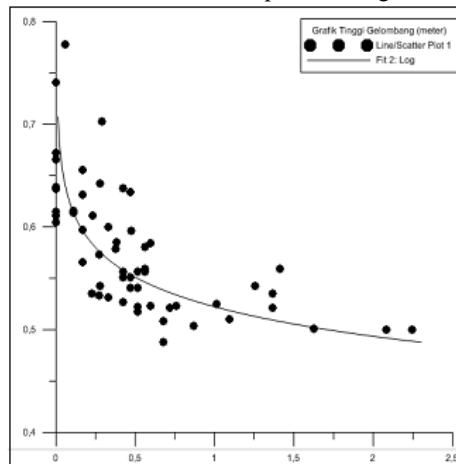
Gambar 7. Hasil fitting data Tinggi gelombang
