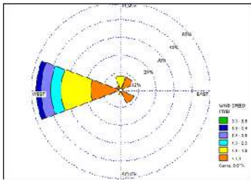
Gambar 3. Windrose musim Barat (2003-2012)
