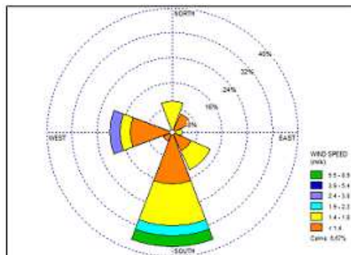
Gambar 5. Windrose musim Timur (2003-2012)
