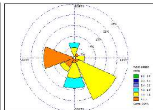
Gambar 6. Windrose musim Peralihan II (2003-2012)
