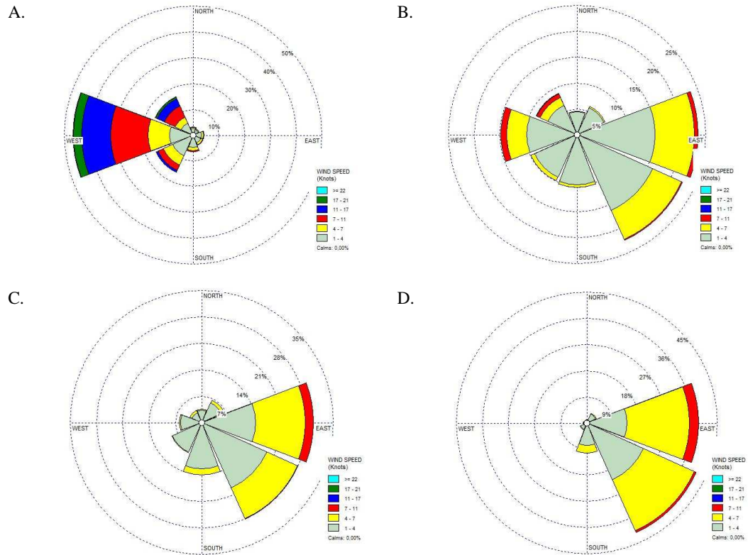
Gambar 4. Wind Rose Gelombang Peramalan Permusim ; A. Musim Barat; B. Musim Peralihan II; C. Musim Timur; D. Musim Peralihan II (Sumber : Pengolahan Data Angin BMKG, 2014).
