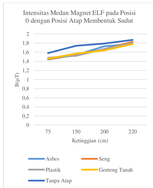
Gambar 3. Pola distribusi intensitas radiasi medan magnet ELF di bawah SUTT 150 kV Sempu-Banyuwangi dengan penghalang atap berbeda pada posisi 0 dengan posisi atap membentuk sudut
