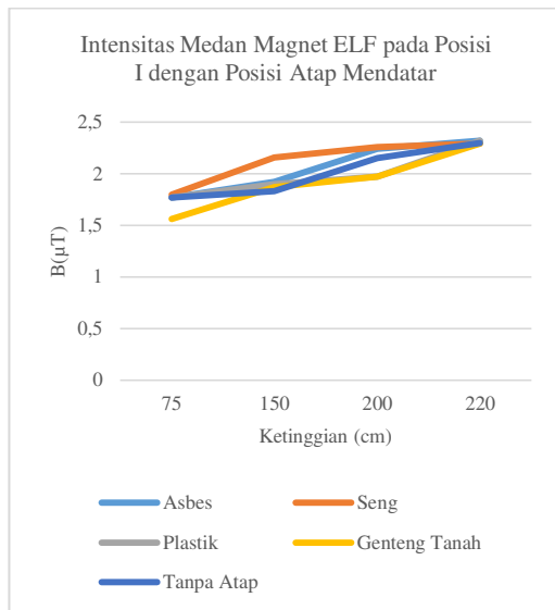
Gambar 4. Pola distribusi intensitas radiasi medan magnet ELF di bawah SUTT 150 kV Sempu-Banyuwangi dengan penghalang atap berbeda pada posisi I dengan posisi atap mendatar
