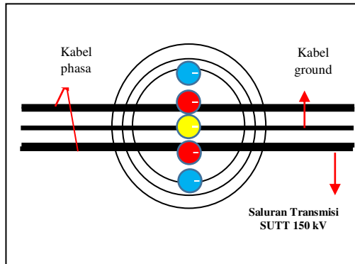
Gambar 1. Sketsa titik-titik pengukuran medan magnet terhadap SUTT 150kV secara lateral tampak atas
