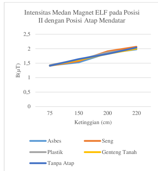
Gambar 6. Pola distribusi intensitas radiasi medan magnet ELF di bawah SUTT 150 kV Sempu-Banyuwangi dengan penghalang atap berbeda pada posisi II dengan posisi atap mendatar
