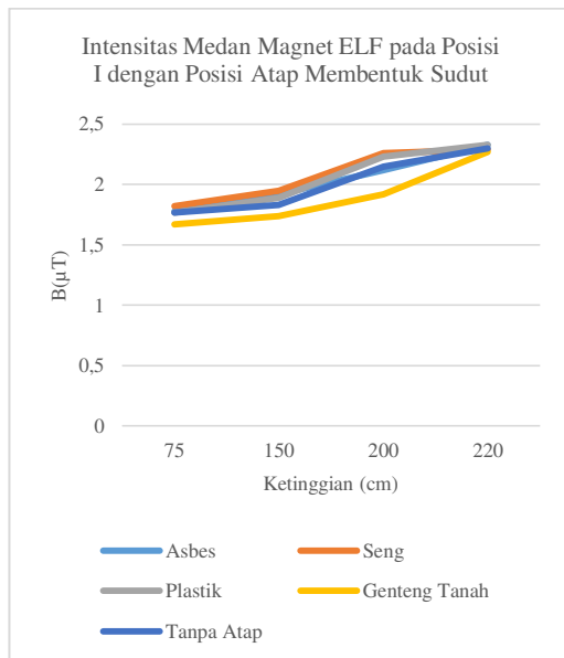
Gambar 5. Pola distribusi intensitas radiasi medan magnet ELF di bawah SUTT 150 kV Sempu-Banyuwangi dengan penghalang atap berbeda pada posisi I dengan posisi atap membentuk sudut
