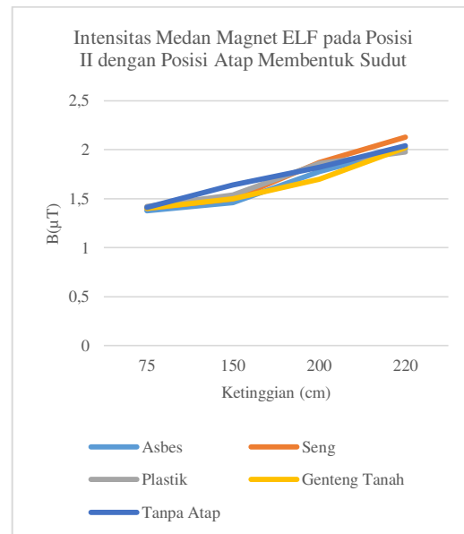
Gambar 7. Pola distribusi intensitas radiasi medan magnet ELF di bawah SUTT 150 kV Sempu-Banyuwangi dengan penghalang atap berbeda pada posisi II dengan posisi atap membentuk sudut
