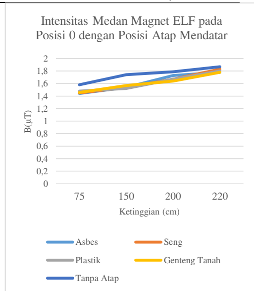
Gambar 2 Pola distribusi intensitas radiasi medan magnet ELF di bawah SUTT 150 kV Sempu-Banyuwangi dengan penghalang atap berbeda pada posisi 0 dengan posisi atap mendatar
