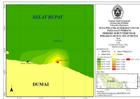
Gambar 7d. Pola air buangan outlet separator-I pada kondisi perbaniperiodesurutterendah diperairanDumaibulanFebruari 2014
