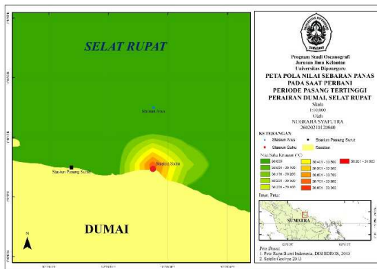
Gambar 7b. Pola air buangan outlet separator-I pada kondisi perban periode pasang tertinggi diperairan Dumaibulan Februari 2014
