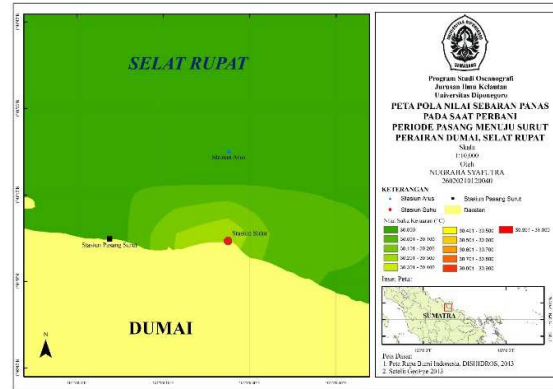
Gambar 7c. Pola air buangan outlet separator-I pada kondisi perbaniperiode pasang menuju surut diperairan Dumaibulan Februari 2014
