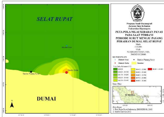
Gambar 7a. Pola air buangan outlet separator-I padakondisiperbaniperiodesurutmenujupasang diperairanDumaibulanFebruari 2014
