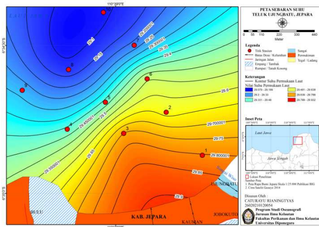
Gambar 3. Peta Sebaran Suhu (°C) di Perairan Teluk Ujungbatu Jepara
