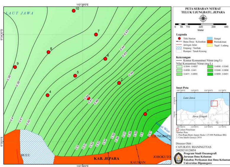
Gambar 1. Peta Sebaran Konsentrasi Nitrat (mg/l) di Perairan Teluk Ujungbatu
