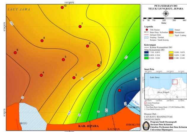
Gambar 5. Peta Sebaran DO (mg/l) di Perairan Teluk Ujungbatu Jepara
