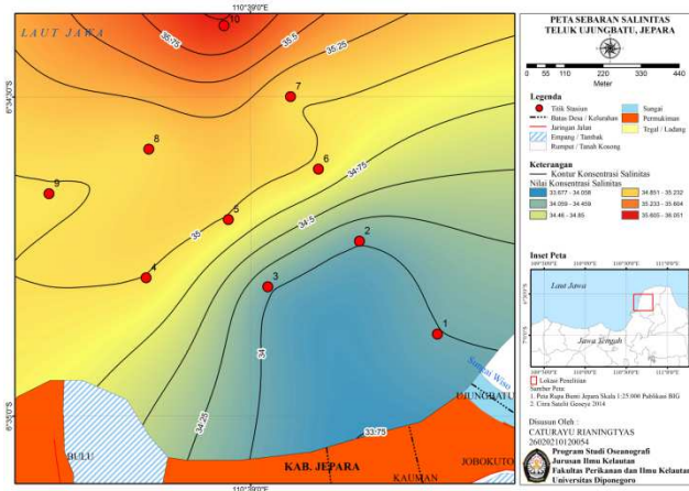
Gambar 4. Peta Sebaran Salinitas (‰) di Perairan Teluk Ujungbatu Jepara
