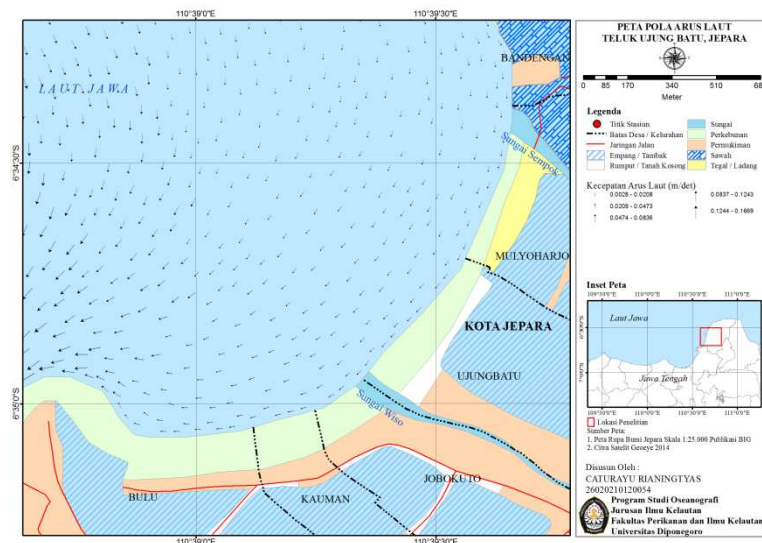
Gambar 6. Peta arah dan pergerakan arus di perairan Teluk Ujungbatu Jepara
