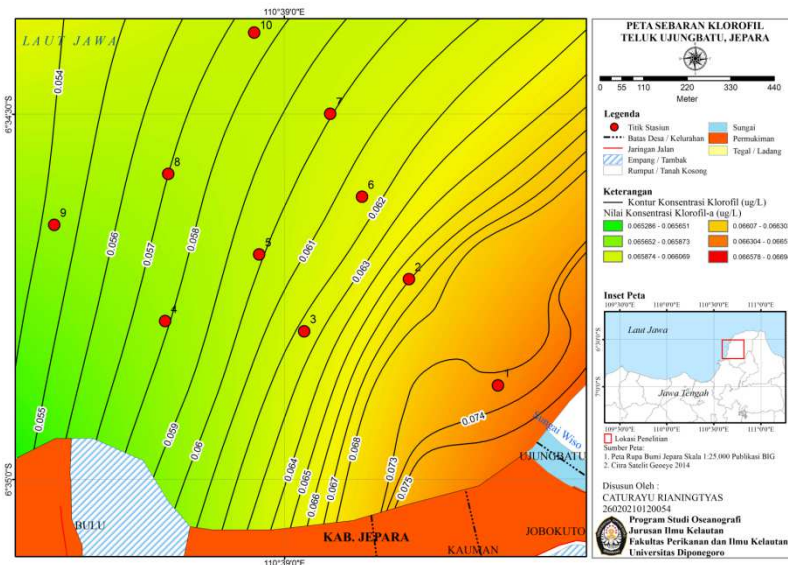
Gambar 2. Peta Sebaran Konsentrasi klorofil-a ( \mu\text{g/l} ) di Perairan Teluk Ujungbatu Jepara
