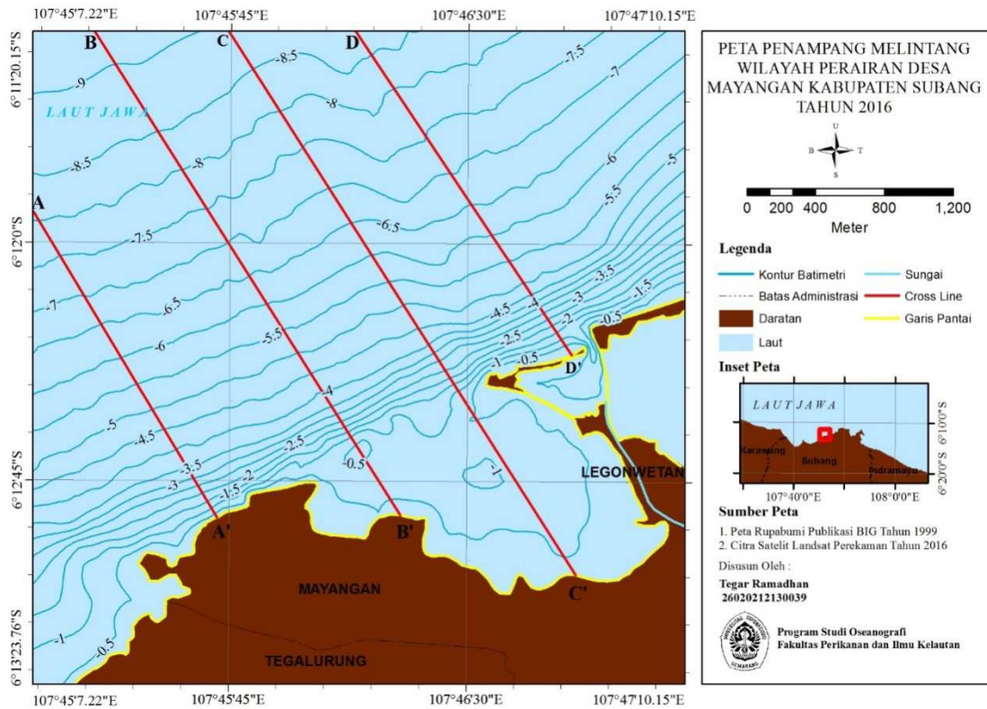
Gambar 6. Peta Penampang Melintang Kedalaman Wilayah Perairan Desa Mayangan, Kabupaten Subang
