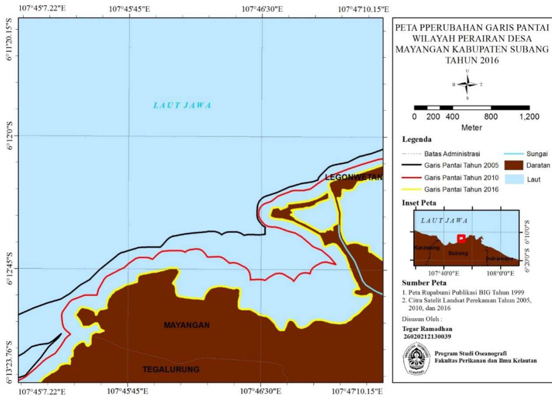
Gambar 12. Peta Perubahan Garis Pantai Wilayah Perairan Desa Mayangan Kabupaten Subang Tahun 2005 – 2016
