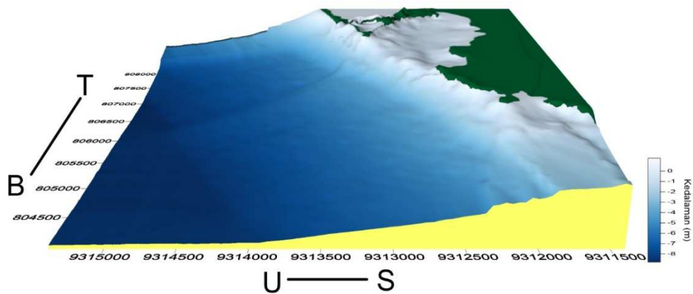
Gambar 5. Model 3D Wilayah Perairan Desa Mayangan, Kabupaten Subang dengan exaggeration 1 : 75
