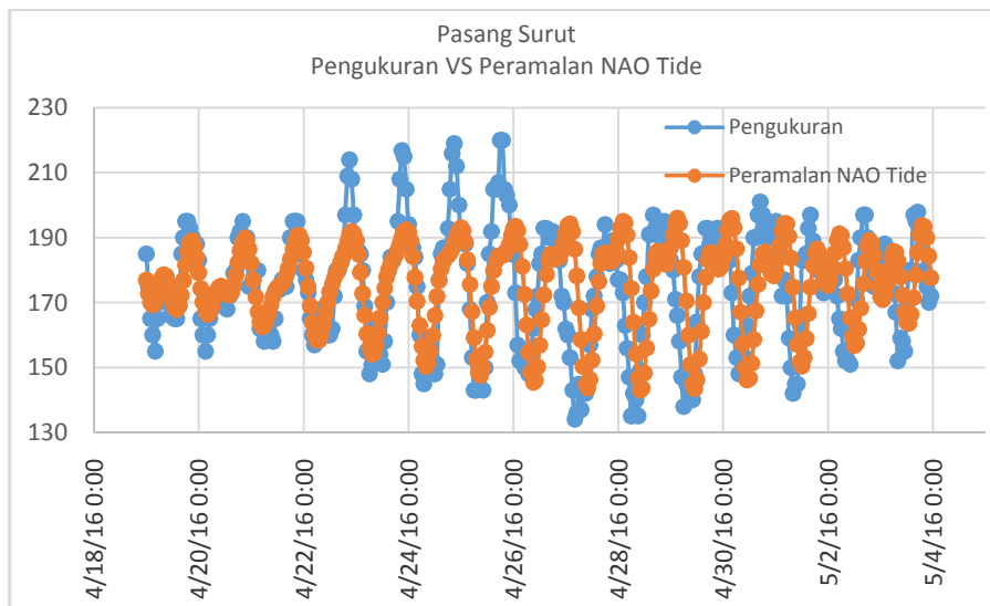
Gambar 1. Grafik Perbandingan Elevasi Pasang Surut Pengukuran dan Peramalan NAO Tide di Lokasi Penelitian
