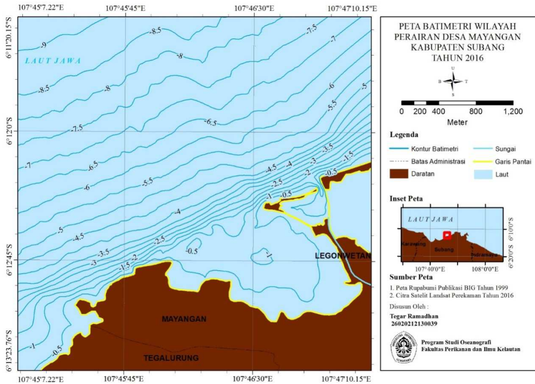
Gambar 4. Peta Batimetri Wilayah Perairan Desa Mayangan, Kabupaten Subang
