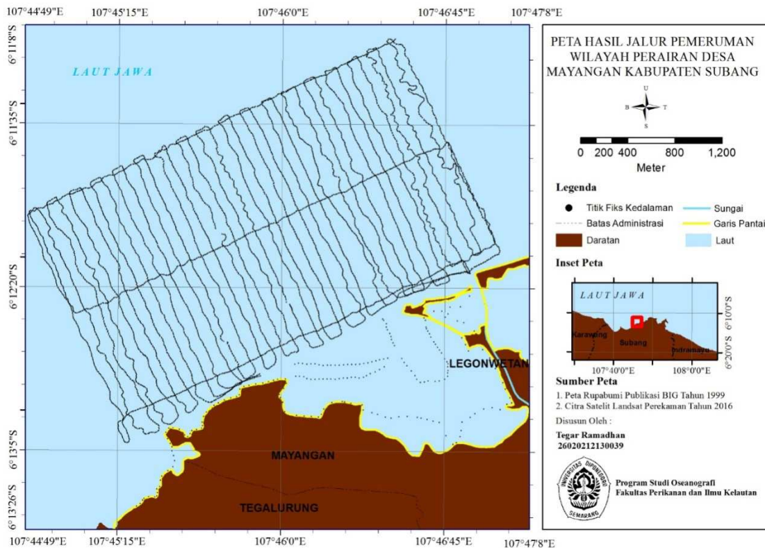
Gambar 3. Hasil Jalur Pemeruman Batimetri Wilayah Perairan Desa Mayangan, Kabupaten Subang
