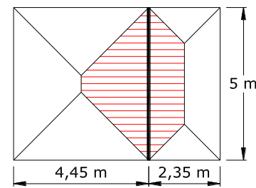
Gambar 9. Beban Amplap pada Balok Anak BA
