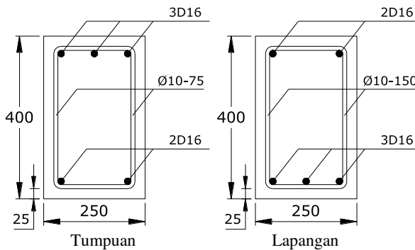
Gambar 6. Potongan Balok Tangga G7C
