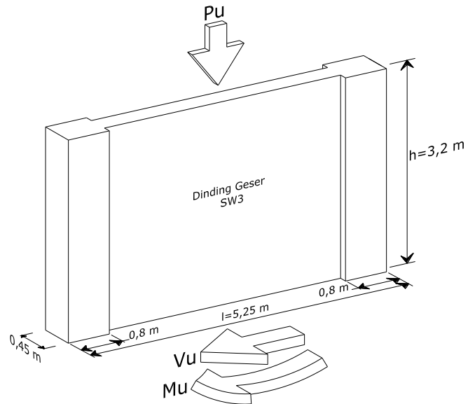
Gambar 22. Gaya-gaya Dalam pada Dinding Geser
