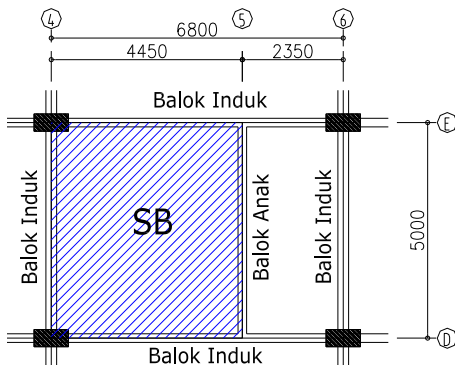
Gambar 7. Denah Pelat Lantai SB Lantai Mezzanine yang Ditinjau
