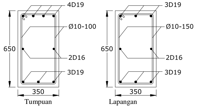
Gambar 17. Penulangan dan Potongan Balok Induk G2A (350x650)
