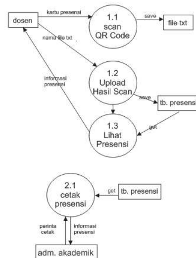
Gambar 5.5. Diagram Level 2 Mesin Presensi Cepat dengan QR Code dan Webcam
