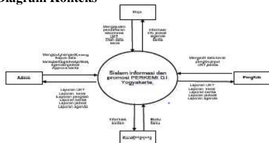
Gambar 3. Diagram Konteks
