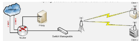
Gambar 1 Topologi Sebelum Pemasangan Server
