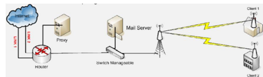
Gambar 2 Topologi Setelah Pemasangan Server
